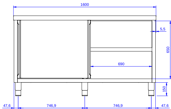
Boční
